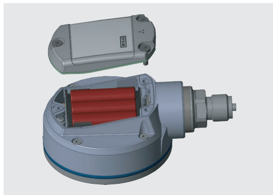
Fig. 1: Posición del compartimento de pilas
